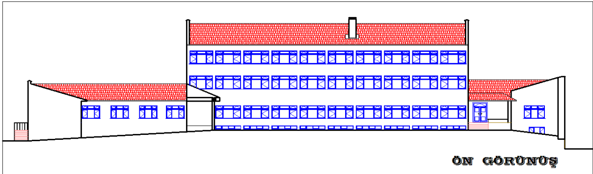
Şekil 2.3 AKML mevcut ön görünüş
