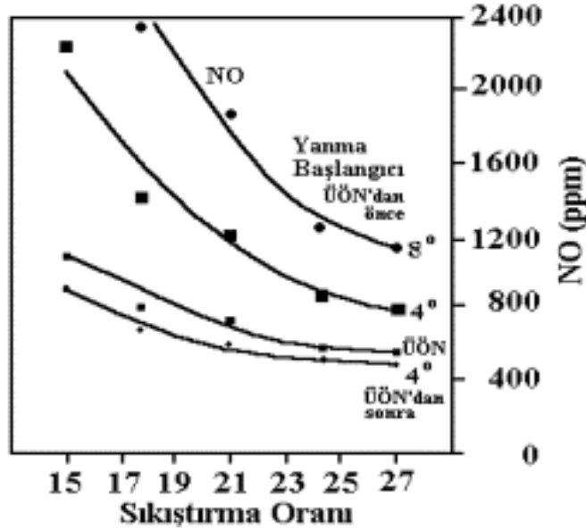
Şekil 12. Sıkıştırma Oranı Değişiminin NO Emisyonlarına Etkisi (36)
