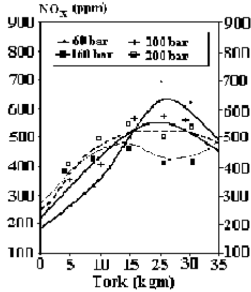
Şekil 8 Değişik Enjektör Püskürtme Basınçlarına Bağlı Olarak NO x Değişimi (30).
