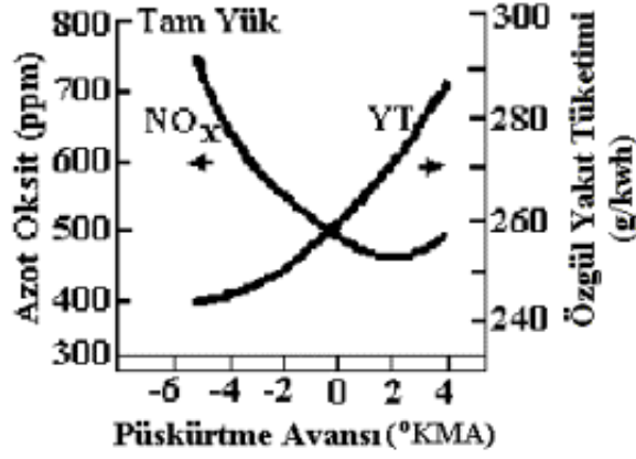
Şekil 7 Püskürtme Avansının NO x ve Yakıt Tüketimine Etkisi (26).
