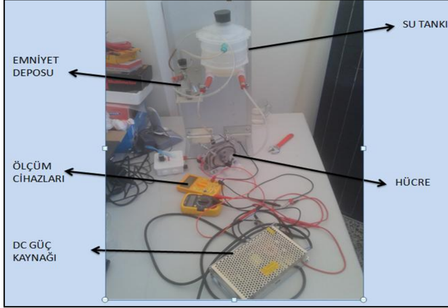
Şekil 2. Deneysel sistem
