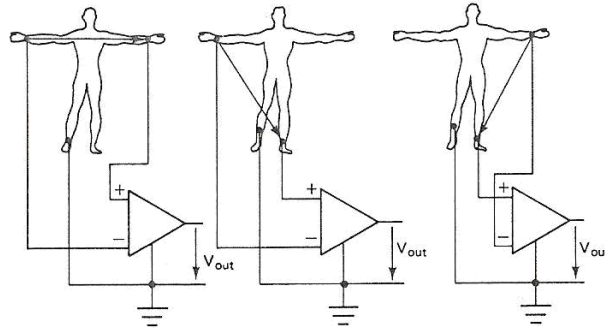
Şekil 3. Bipolar bağlantılar [10]
